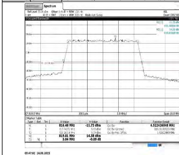
B26(814-824)-10MHz-QPSK-26740-50RB#0-PASS
