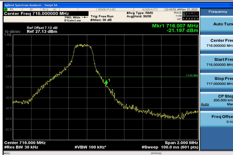
Band12-3MHz-QPSK-23165-1RB#14
