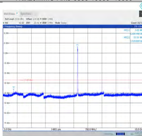
11ax20MIMO-Ant7-6695-3000~10000
