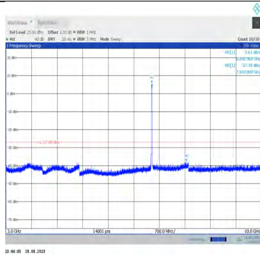
11ax20MIMO-Ant7-6995-3000~10000
