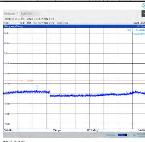
11ax20MIMO-Ant9-7115-30~3000
