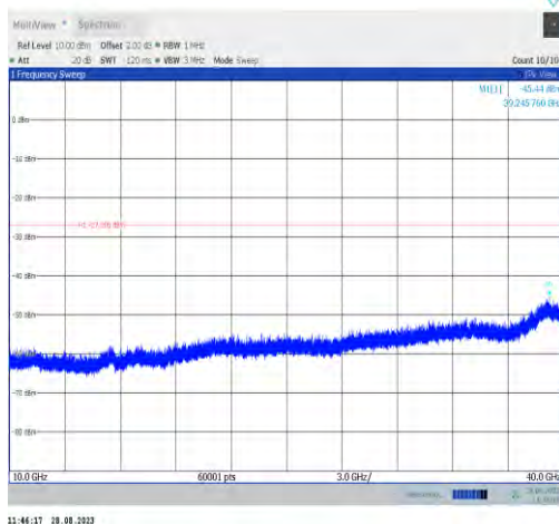
11ax20MIMO-Ant7-6475-10000~40000
