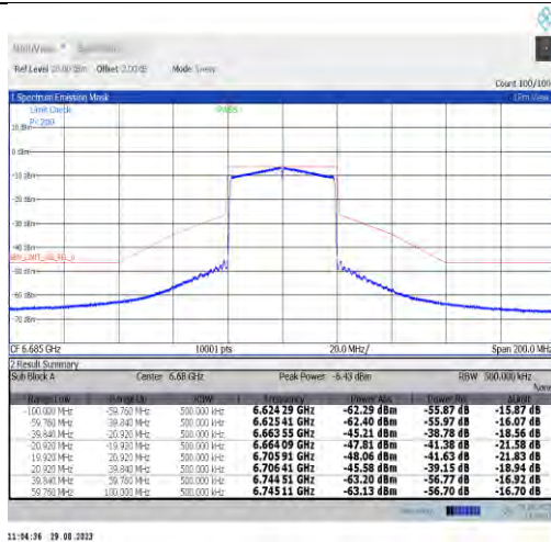
NTNV-11ax40MIMO-Ant7-6685-PASS
