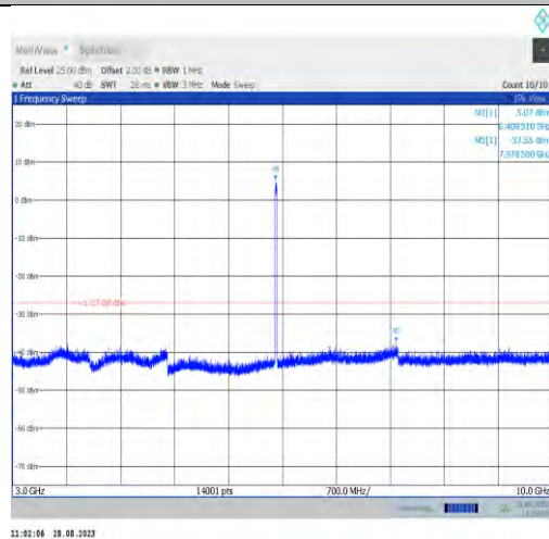
11ax20MIMO-Ant7-6415-3000~10000
