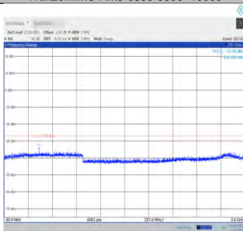
11ax20MIMO-Ant7-6695-30~3000
