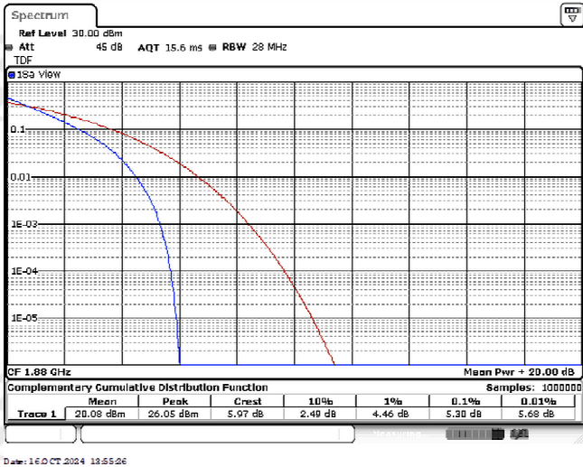
Band2-10MHz-QPSK-18900-50RB#0
