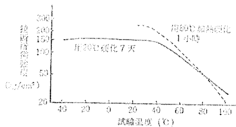
圖 II 2.5 耐熱特性 硬化劑混合率爲 100phr
