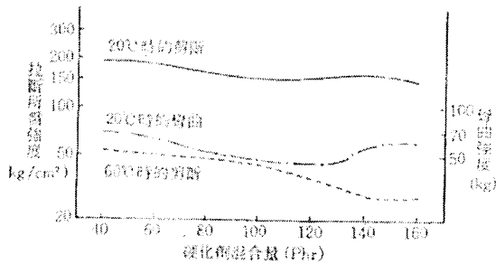
圖 II 2.1 硬化劑混合量と粘着力強度 (在20°C七天の硬化) 試験片：鉄鋼板 (25×100×1.6mm) (Over-lap)12.5mm
