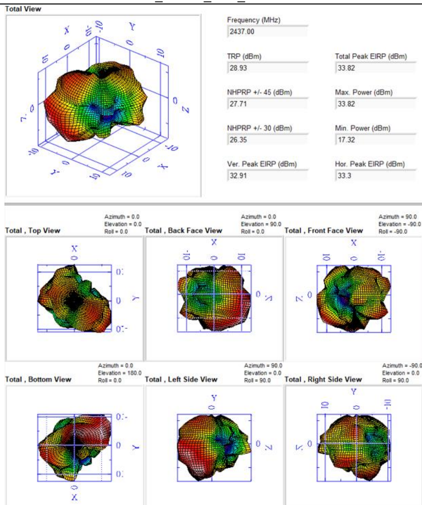
2.4GHz_EHT20_CH6_BF On Nss1
