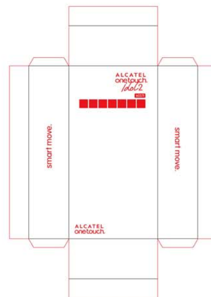
bottom side 179*92*41.5mm
