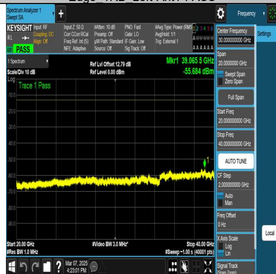
NTNV-N77-3700-3980-PC2-30-20-L-DFT-QPSK- Edge 1RB Left-Ant1-PASS
