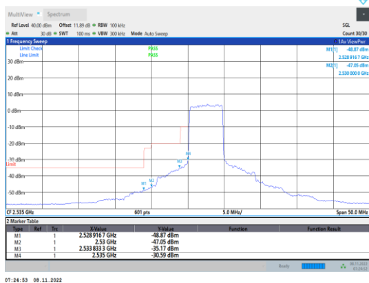
Band41-5MHz-QPSK-40065-25RB#0
