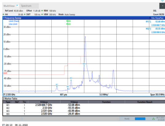
Band41-5MHz-QPSK-40065-1RB#0
