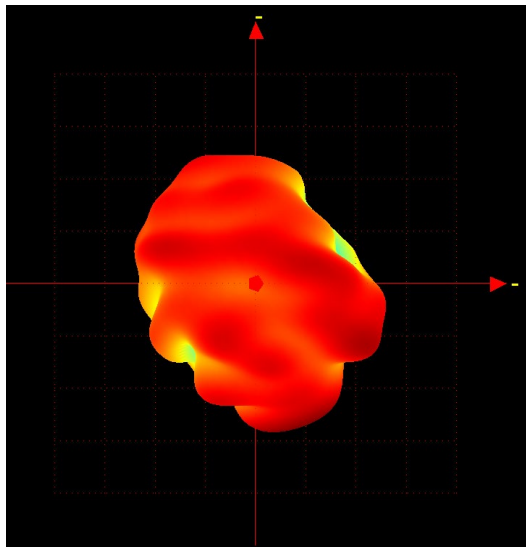
Y 2440MHz
