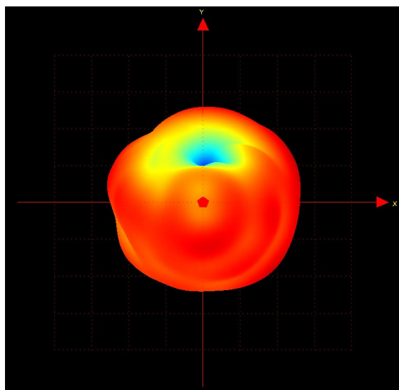
Z 2440MHz
