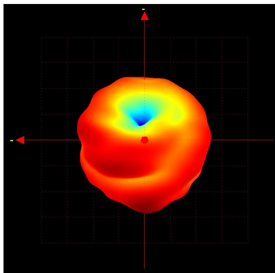
Z 2440MHz
