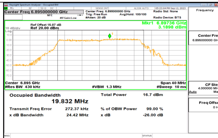
11BE20MIMO_Ant3_6895
