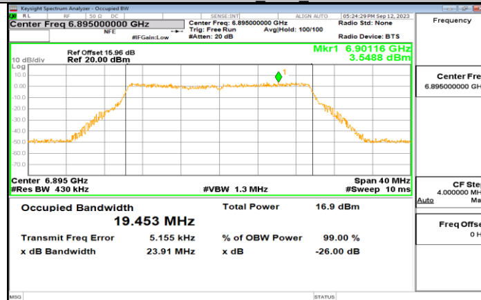
11BE20MIMO Ant4 6895
