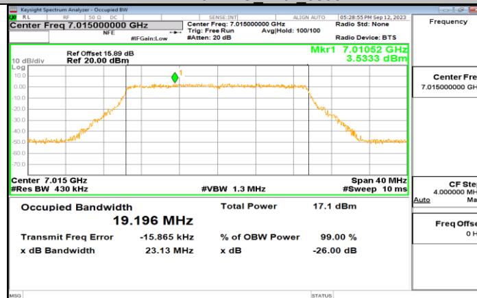
11BE20MIMO Ant1 7015
