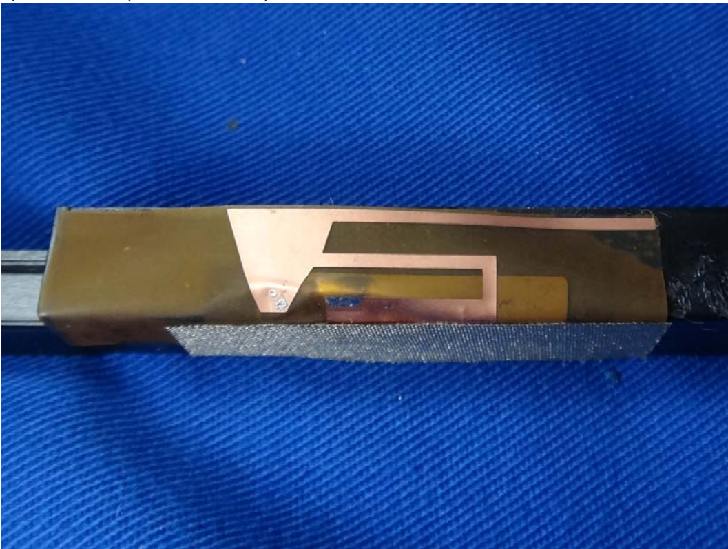
(18) EUT Photo (Antenna-ACON)
