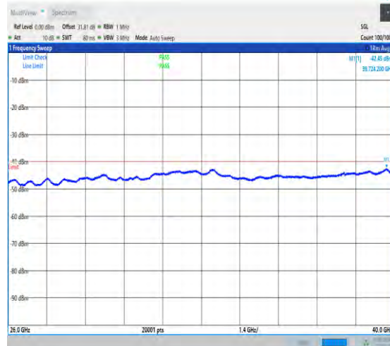
NTVN_N48_PC3_30_40_M_TID1_NS_01_26000_40000_#
