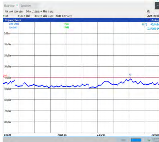
NTVN_N48_PC3_30_40_L_TID1_NS_01_6000_26000_#1
