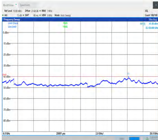
NTVN_N48_PC3_30_40_M_TID1_NS_01_6000_26000_#
