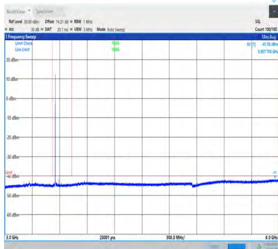
NTVN_N48_PC3_30_40_L_TID1_NS_01_3000_6000_#1
