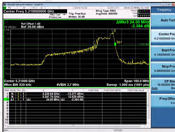
11AX80SISO-Ant1-5210-52Tone-RU52
