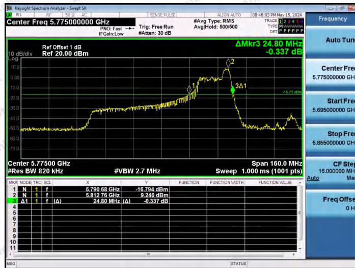
11AX80SISO-Ant1-5775-52Tone-RU52
