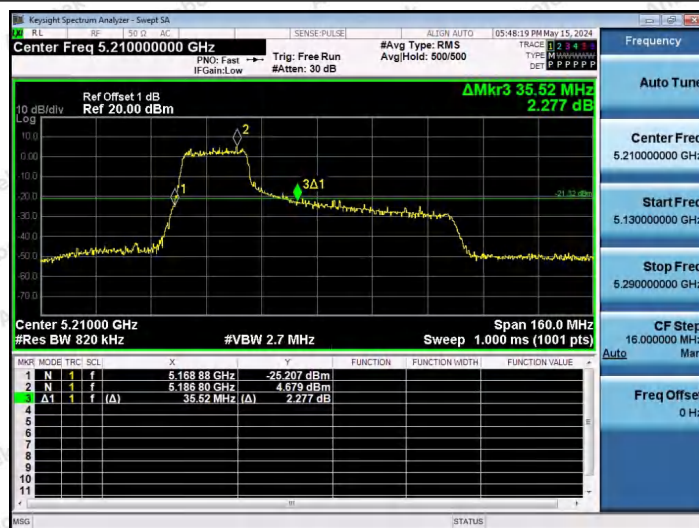
11AX80SISO-Ant1-5210-242Tone-RU61
