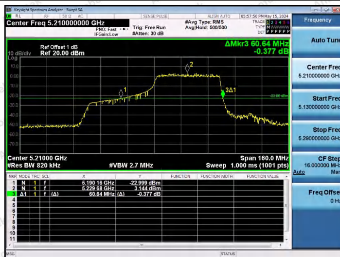
11AX80SISO-Ant1-5210-484Tone-RU66
