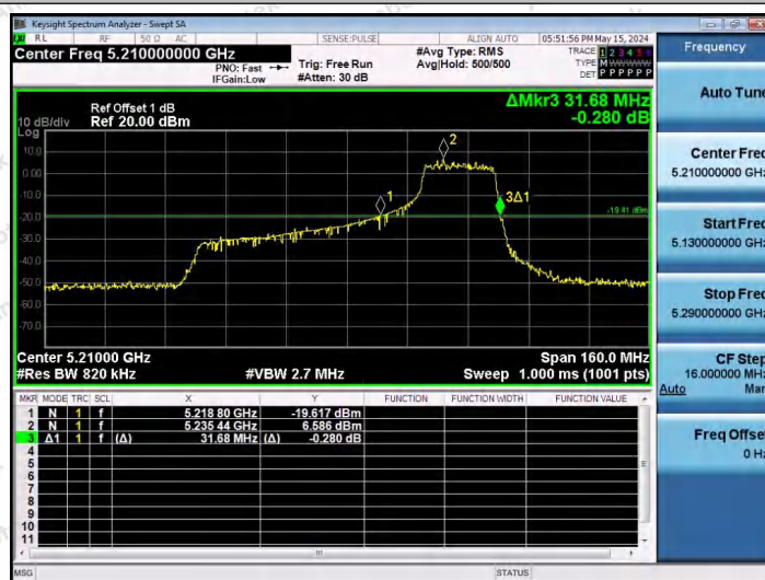
11AX80SISO-Ant1-5210-242Tone-RU64
