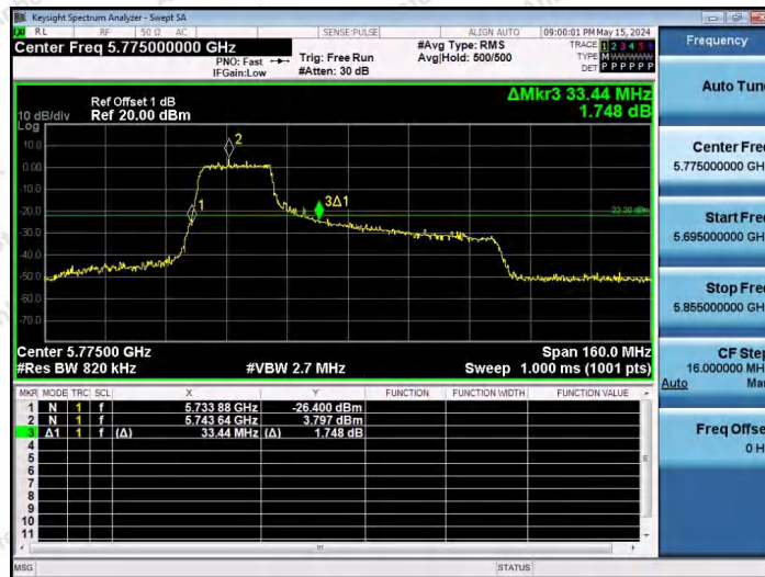
11AX80SISO-Ant1-5775-242Tone-RU61
