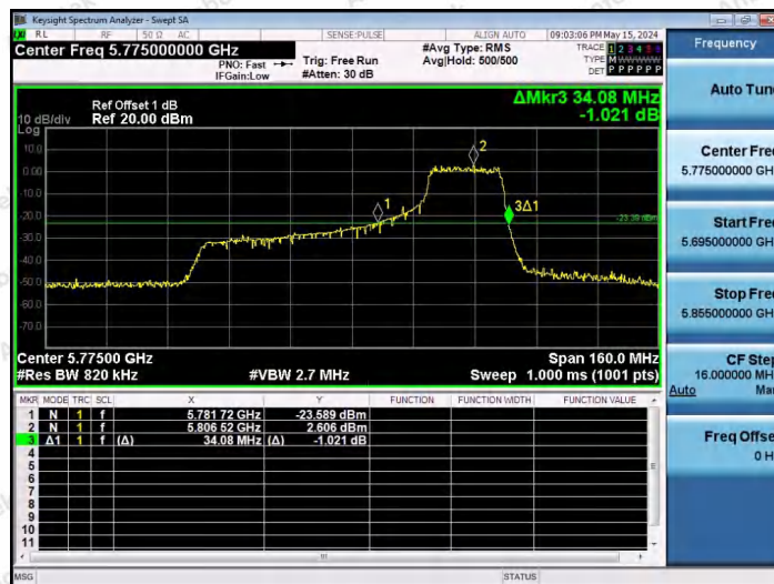
11AX80SISO-Ant1-5775-242Tone-RU64
