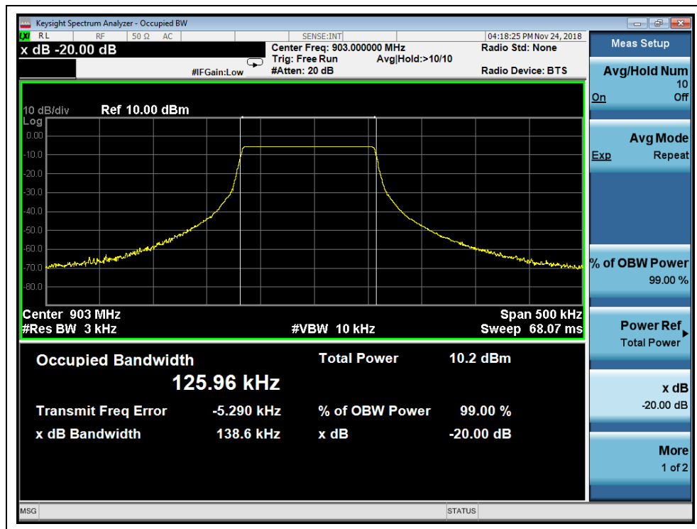
(Channel 1, 903MHz)
