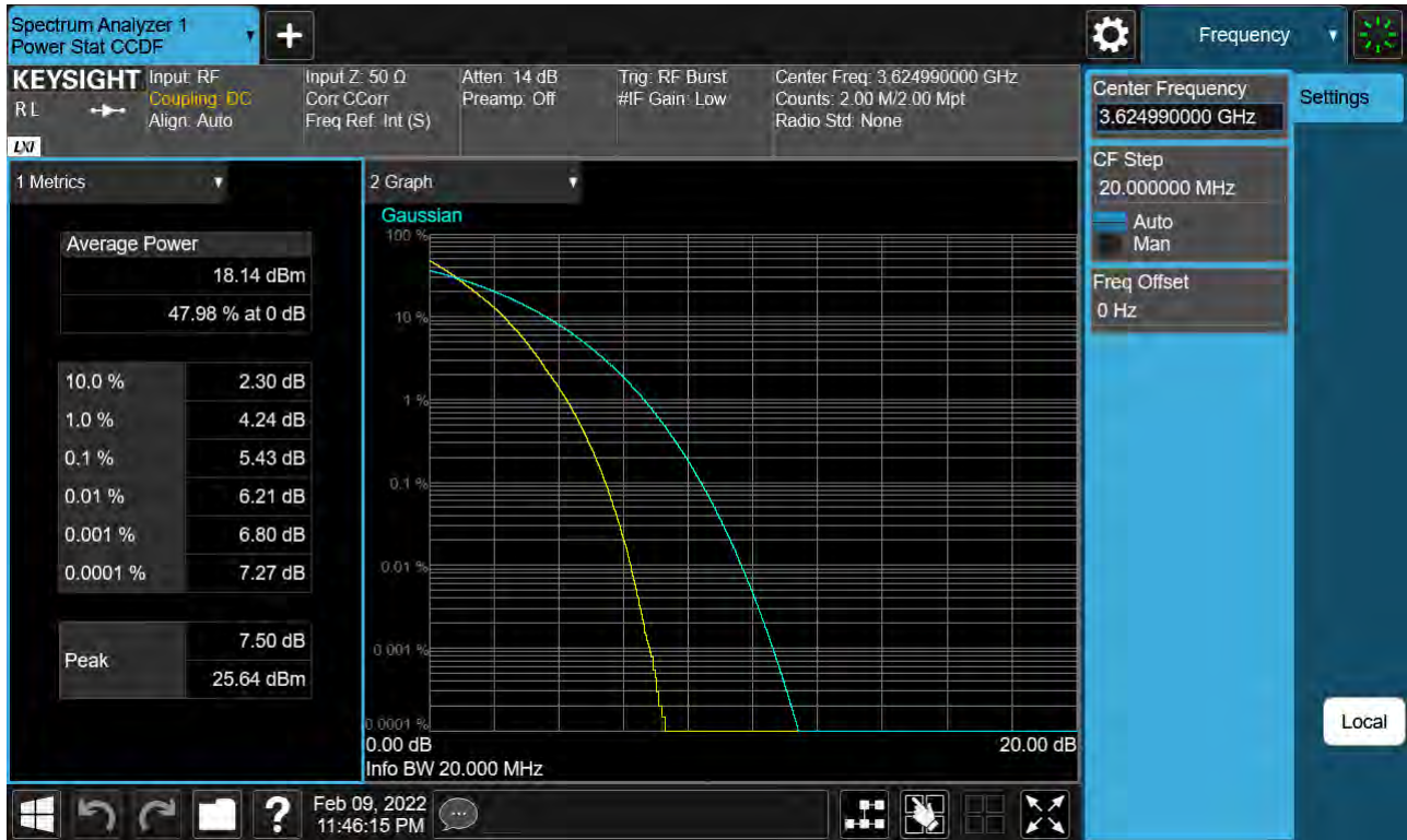
Sub6 n48. PAR Plot (20 MHz Ch. 641666 QPSK)
