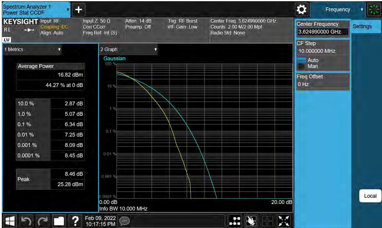
Sub6 n48. PAR Plot (10 MHz Ch.641666 64-QAM)
