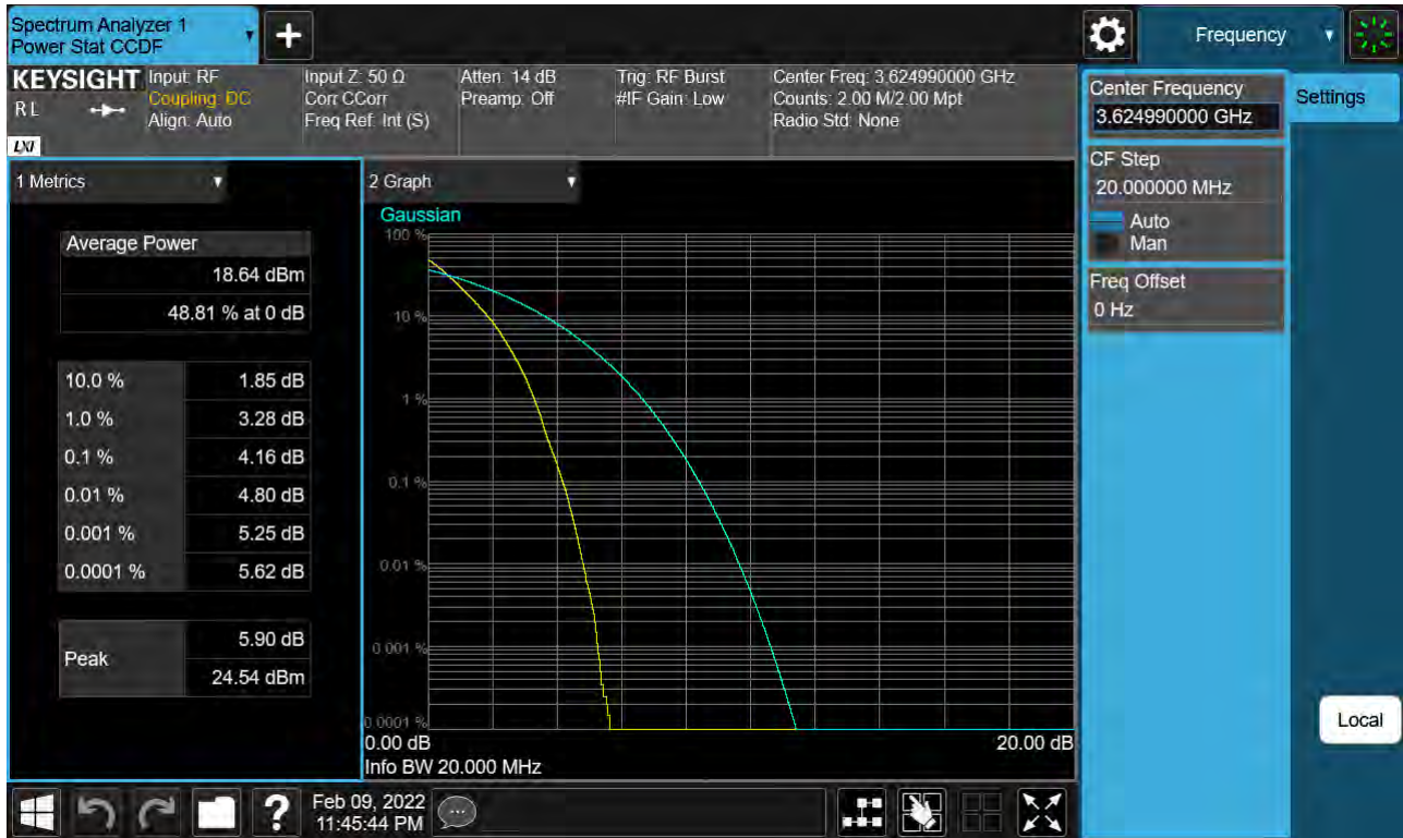
Sub6 n48. PAR Plot (20 MHz Ch. 641666 BPSK)
