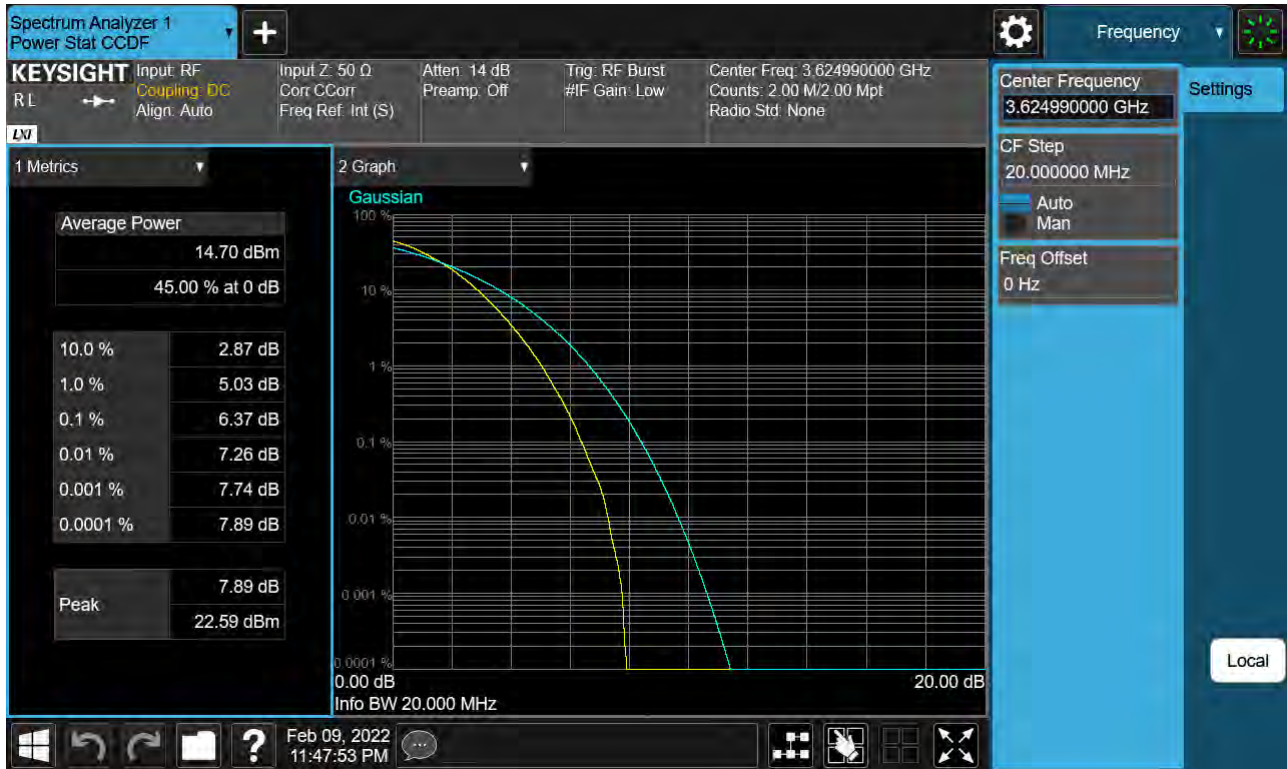
Sub6 n48. PAR Plot (20 MHz Ch.641666 256-QAM)
