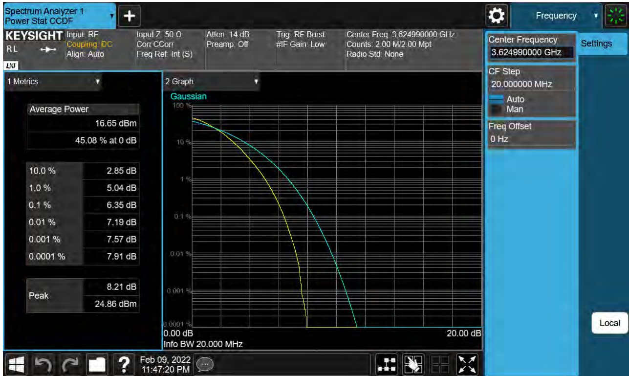
Sub6 n48. PAR Plot (20 MHz Ch.641666 64-QAM)
