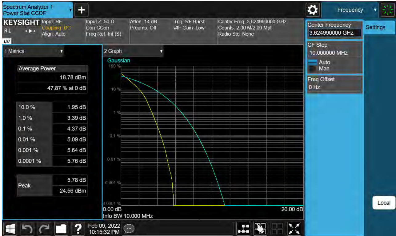
Sub6 n48. PAR Plot (10 MHz Ch. 641666 BPSK)
