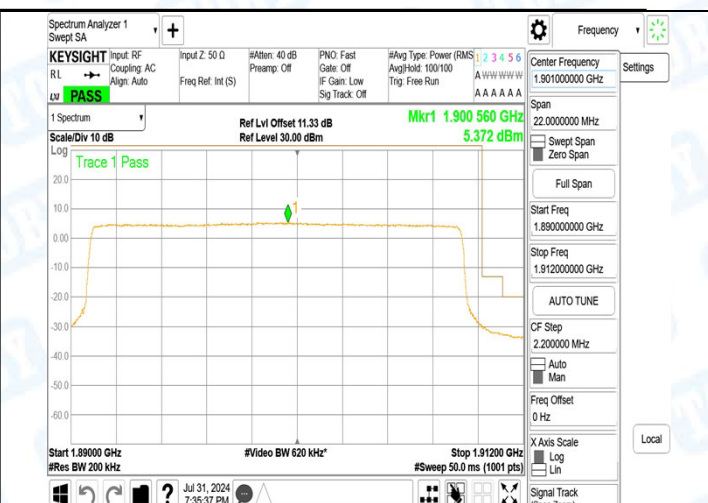
Band2 20MHz 16QAM 18700 1RB#99
