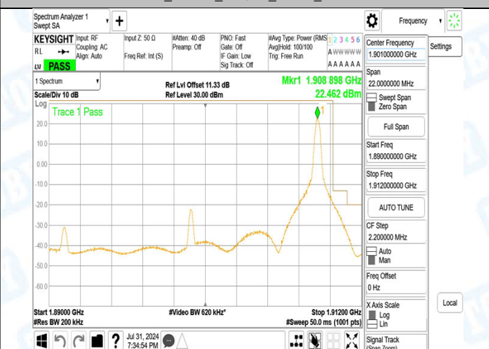
Band2 20MHz 16QAM 19100 1RB#99
