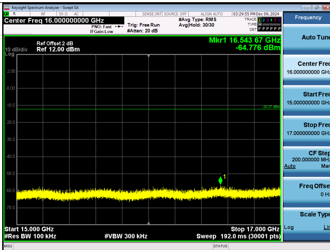
11B-Ant1-2462-15000~17000-PASS
