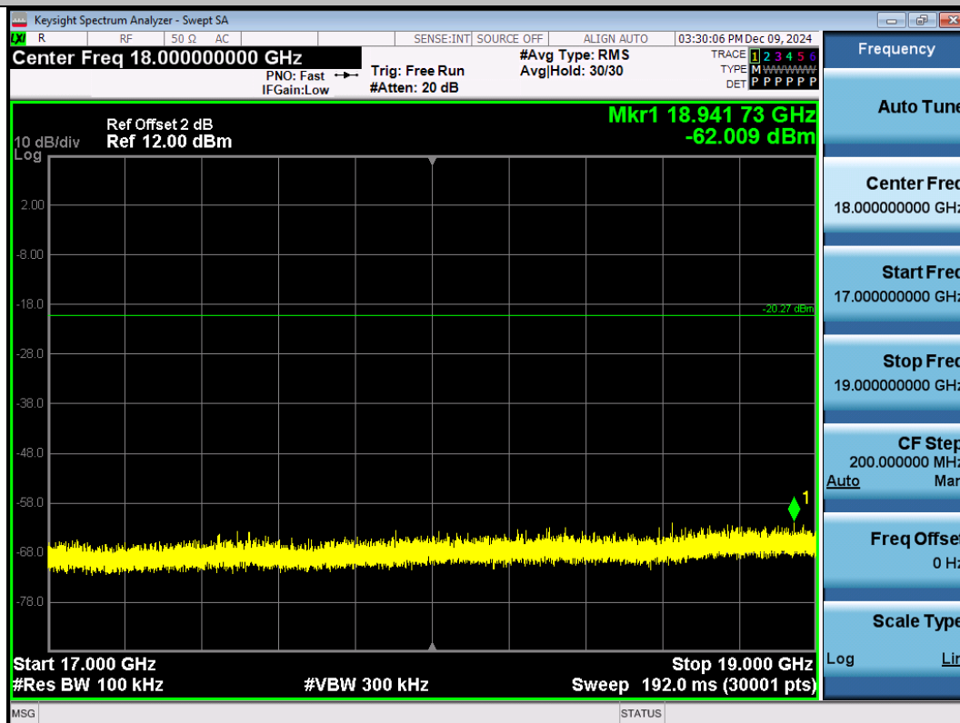
11B-Ant1-2462-17000~19000-PASS
