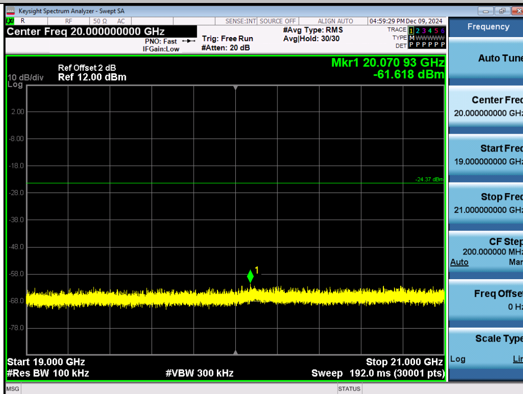
11G-Ant1-2462-19000~21000-PASS
