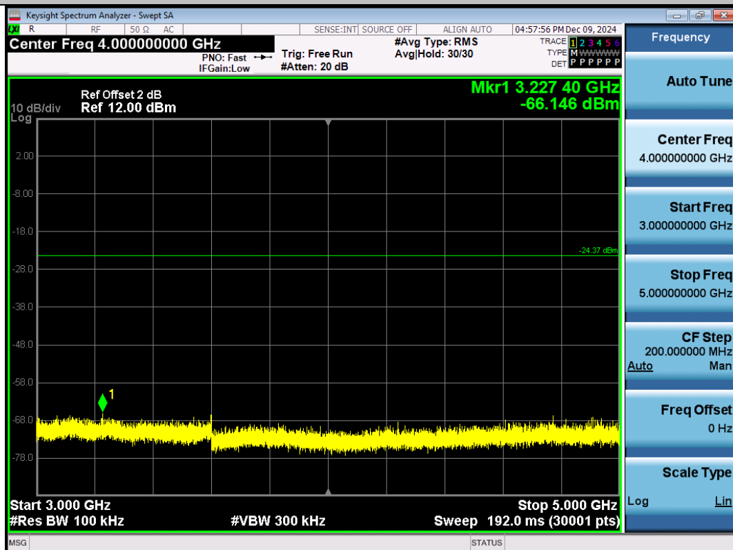
11G-Ant1-2462-3000~5000-PASS
