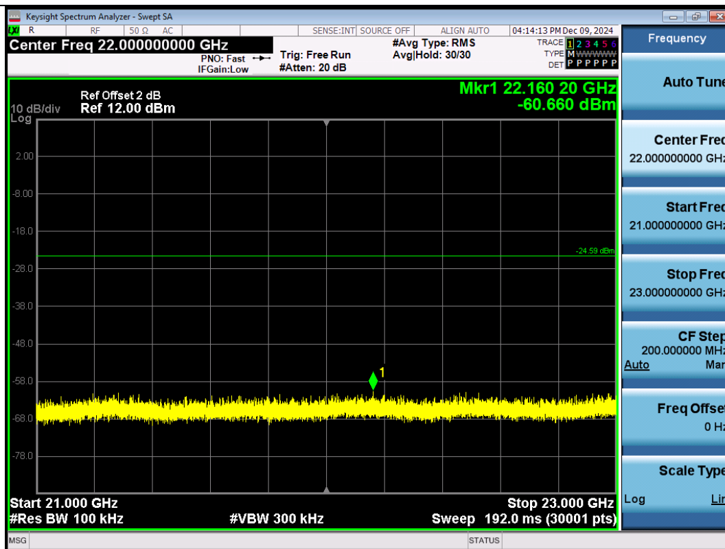
11G-Ant1-2412-21000~23000-PASS
