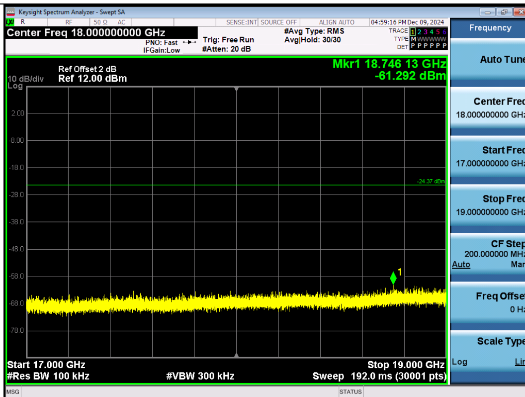
11G-Ant1-2462-17000~19000-PASS
