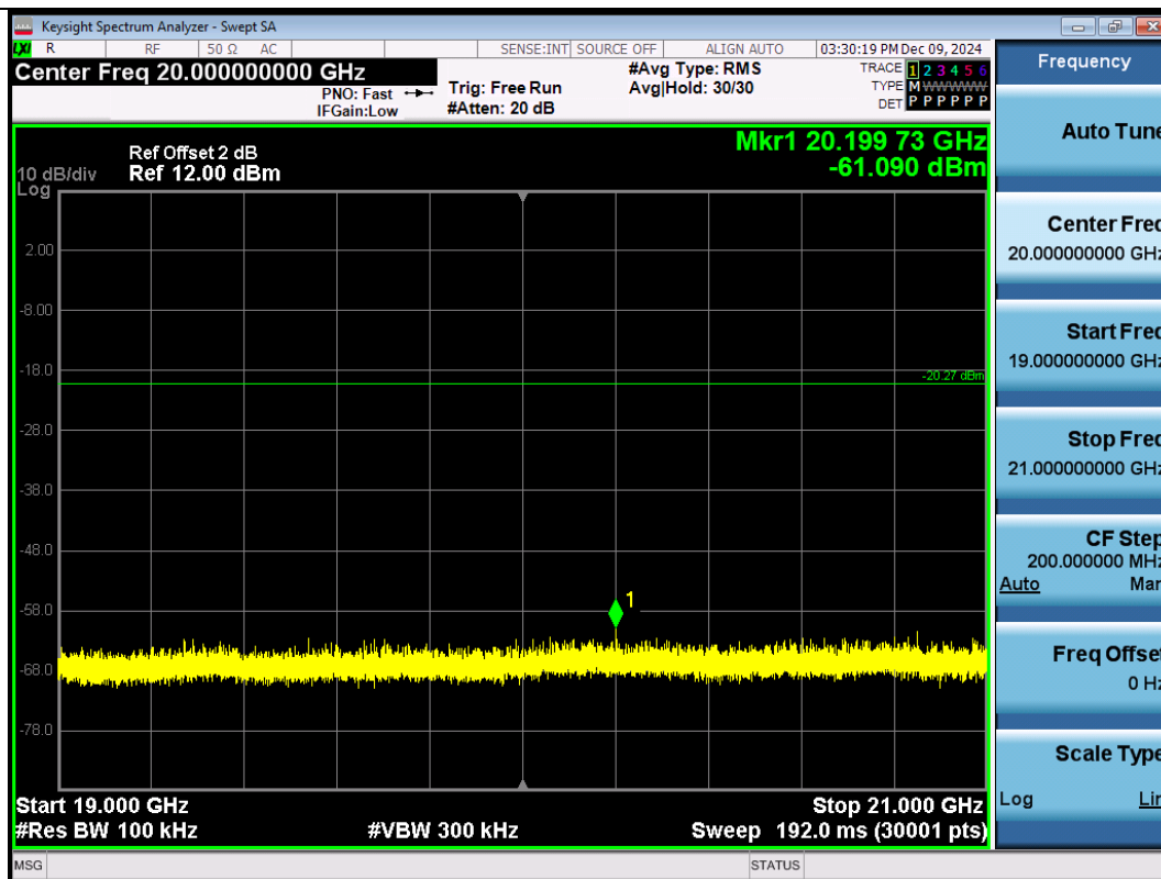
11B-Ant1-2462-19000~21000-PASS
