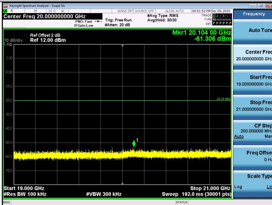
11N40SISO-Ant1-2422-19000~21000-PASS
