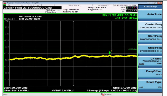
Band41_15MHz_QPSK_41165_75RB#0_20000~27000_20000~27000
