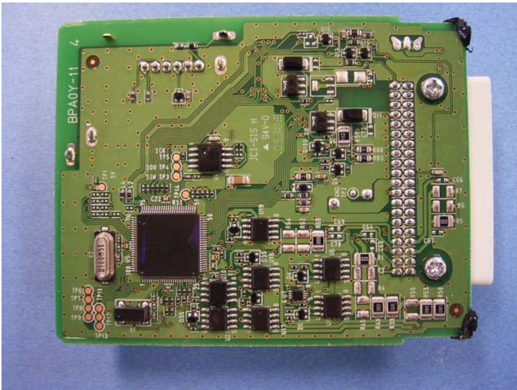
PCB Bottom
