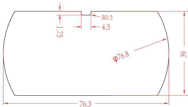
结构尺寸图
