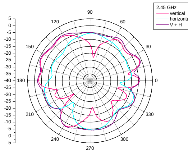
Right antenna open(Aux)
