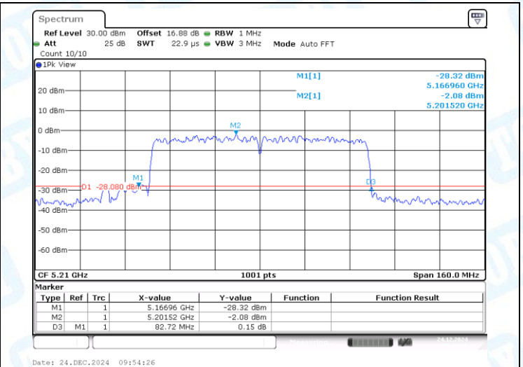
11AC80SISO-Ant1-5210
