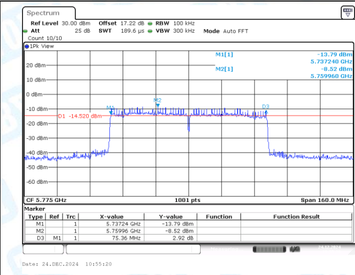
11AC80SISO-Ant1-5775-PASS
