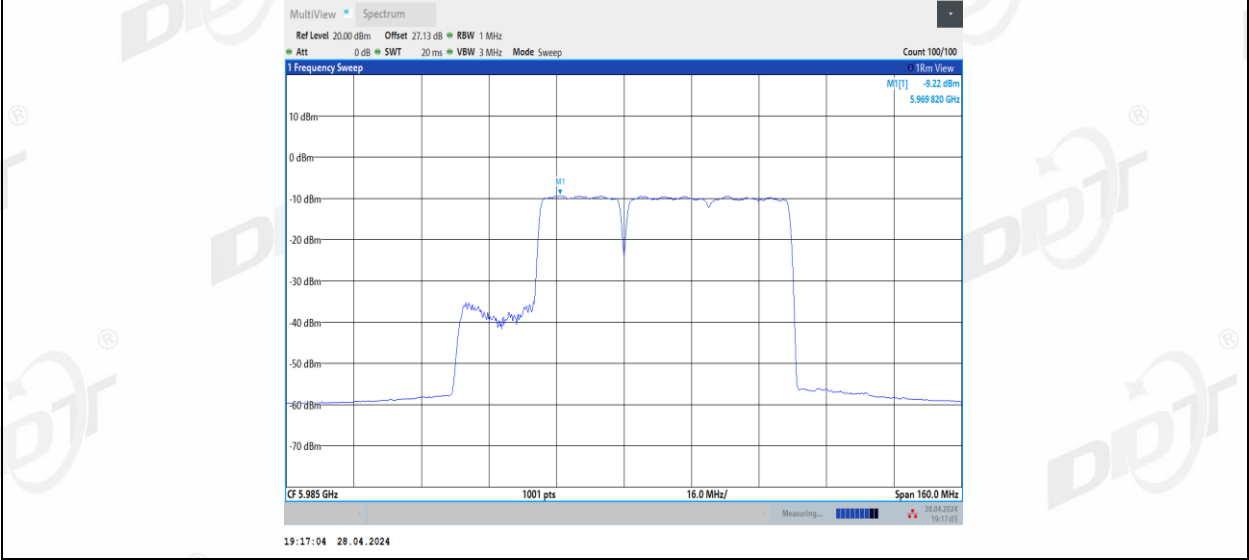
11BE80MIMO_Ant3_5985_484+242_2
