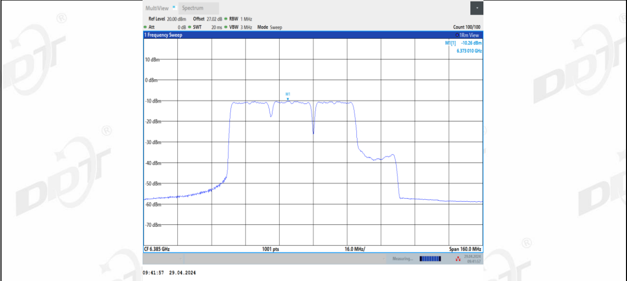
11BE80MIMO_Ant3_6385_484+242_1
