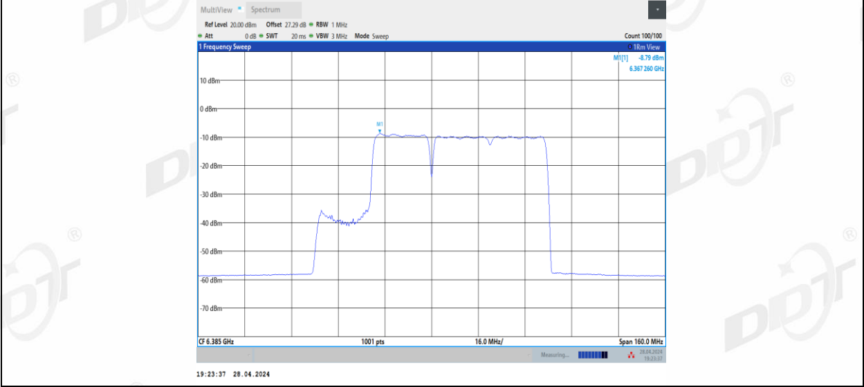
11BE80MIMO_Ant3_6385_484+242_2
