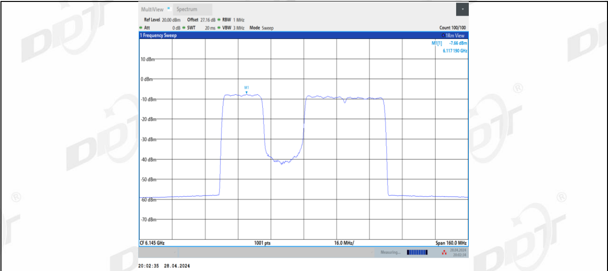
11BE80MIMO_Ant3 6145_484+242_3
