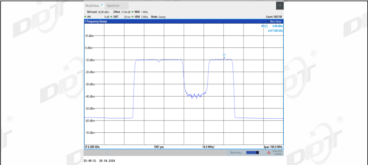
11BE80MIMO_Ant2_6385_484+242_4
