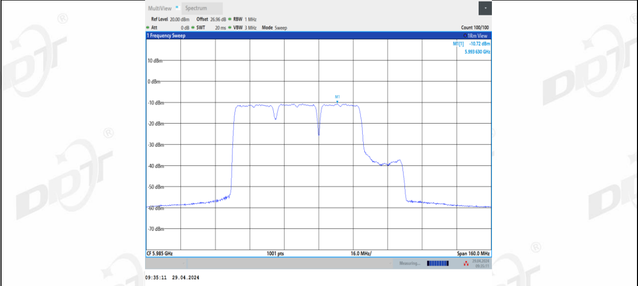
11BE80MIMO_Ant3_5985_484+242_1
