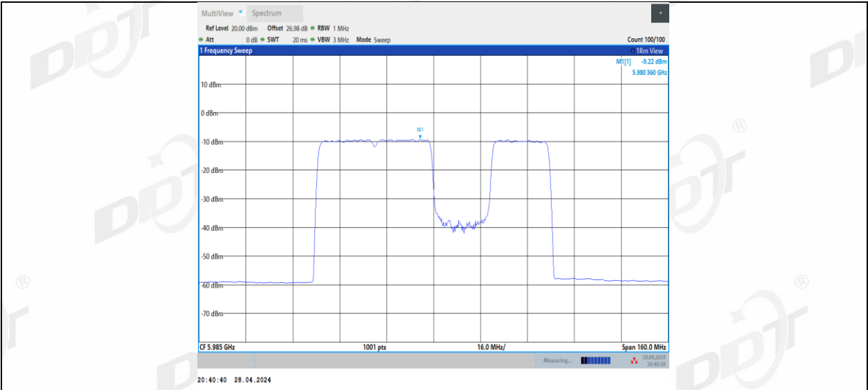
11BE80MIMO_Ant2_5985_484+242_4
