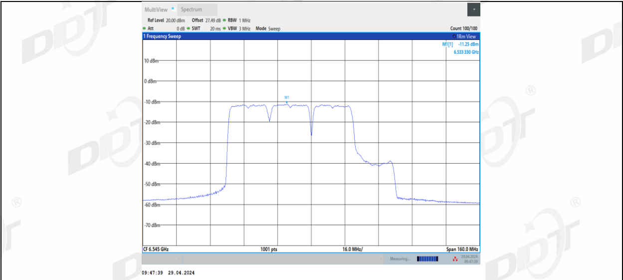
11BE80MIMO_Ant2_6545_484+242_1
