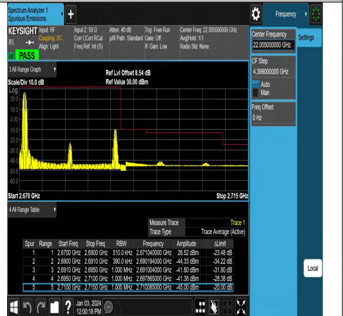
Band41_20MHz_QPSK_41490_1RB#0
