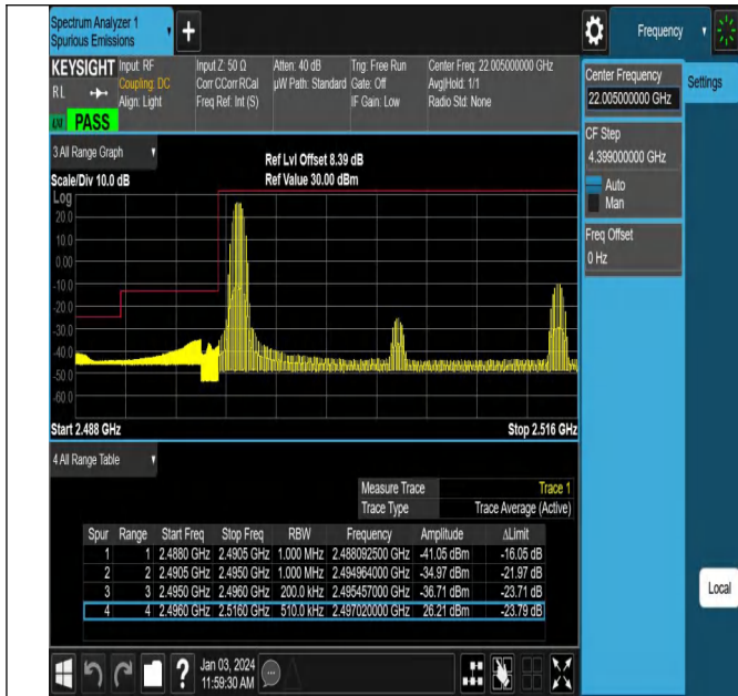
Band41_20MHz_QPSK_39750_1RB#0
