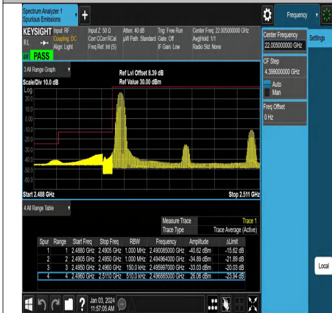
Band41_15MHz_QPSK_39725_1RB#0
