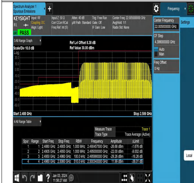
Band41_10MHz_QPSK_39700_50RB#0
