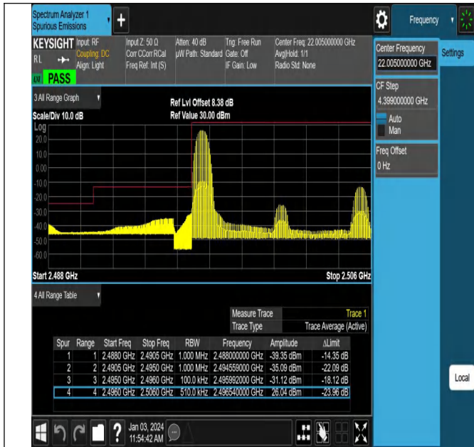
Band41_10MHz_QPSK_39700_1RB#0
