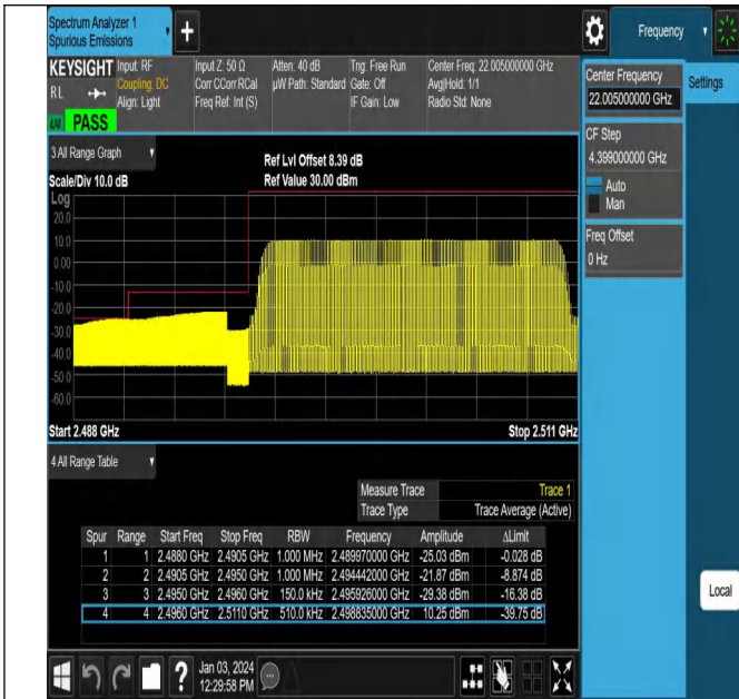
Band41_15MHz_QPSK_39725_75RB#0
