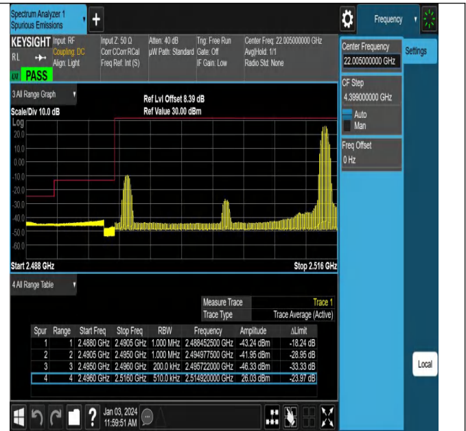
Band41_20MHz_QPSK_39750_1RB#99
