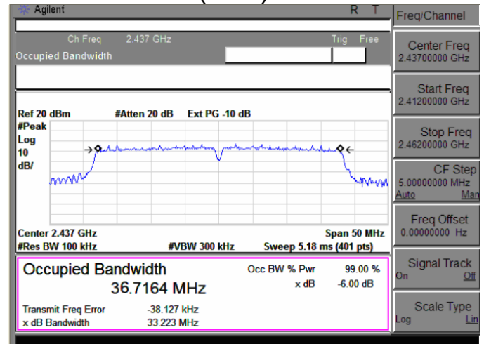
802.11n (HT40) 2437MHz
