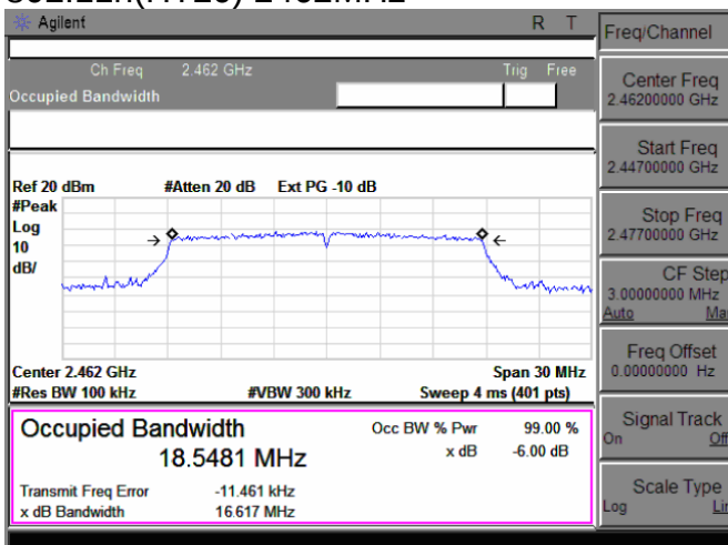
802.11n(HT20) 2462MHz
