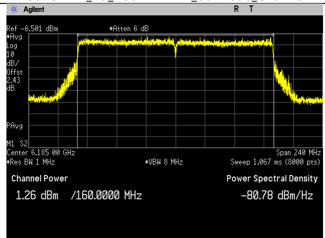
6185MHz_47_160MHz BW_be-mode_Chain 1
