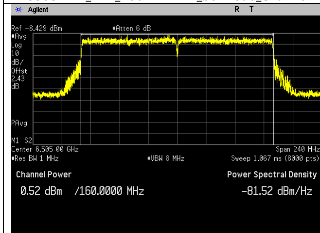
6505MHz_111_160MHz BW_be-mode_Chain 2
