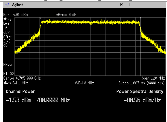
6705MHz_151_80MHz BW_be-mode_Chain 3
