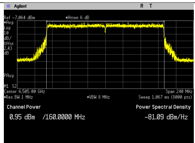
6505MHz_111_160MHz BW_be-mode_Chain 1
