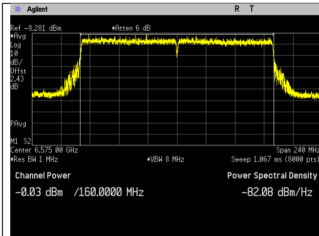
6575MHz_143_160MHz BW_be-mode_Chain 2
