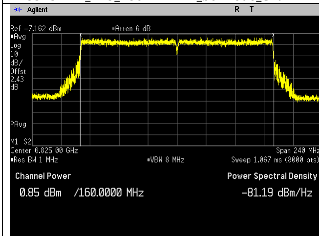
6825MHz_175_160MHz BW_be-mode_Chain 0
