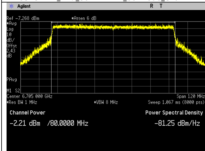
6705MHz_151_80MHz BW_be-mode_Chain 0
