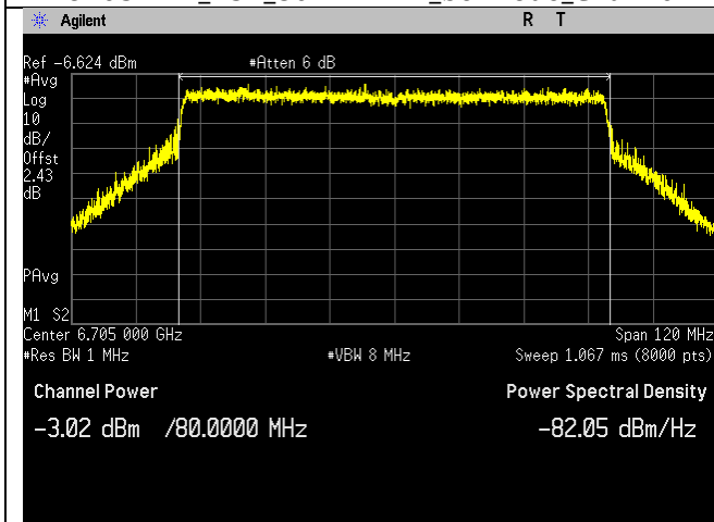
6705MHz_151_80MHz BW_be-mode_Chain 2
