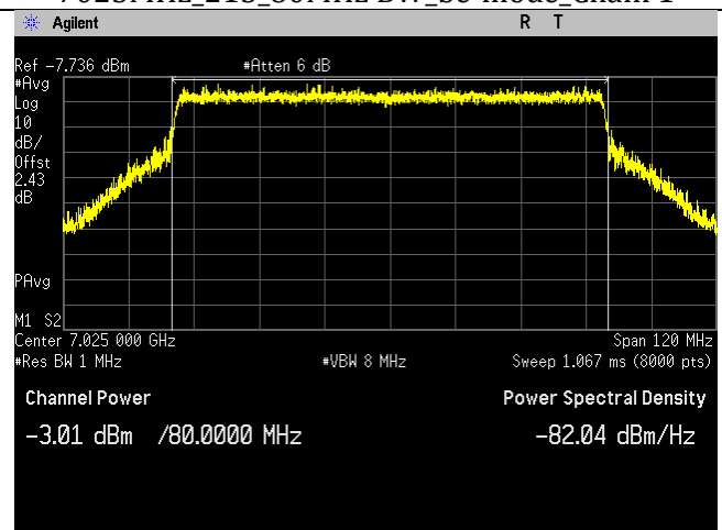
7025MHz_215_80MHz BW_be-mode_Chain 3
