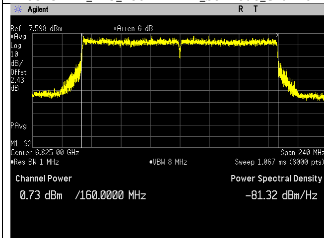
6825MHz_175_160MHz BW_be-mode_Chain 2
