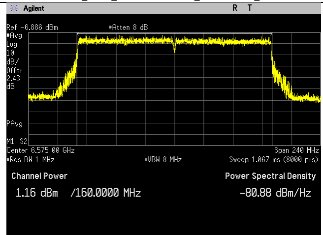
6575MHz_143_160MHz BW_be-mode_Chain 1
