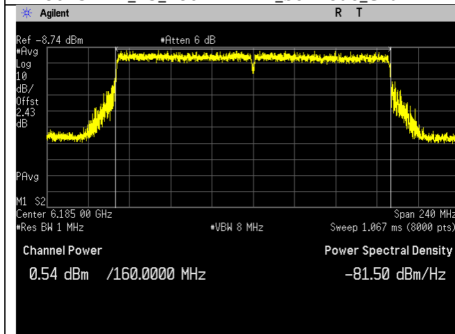
6185MHz_47_160MHz BW_be-mode_Chain 0
