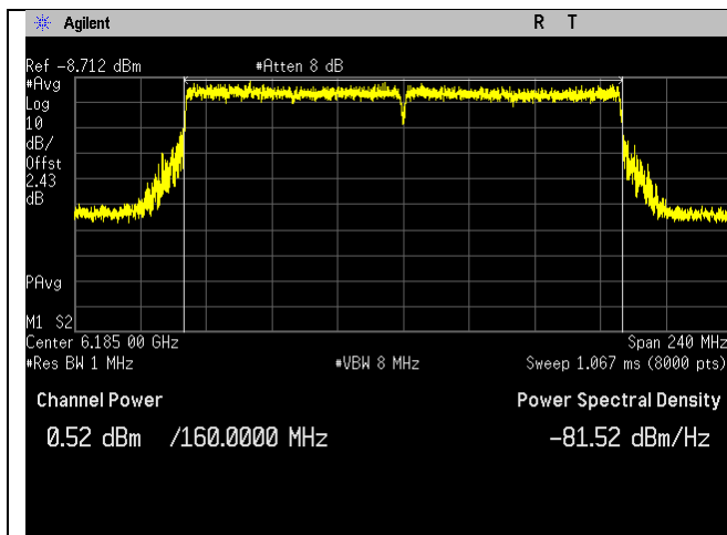
6185MHz_47_160MHz BW_be-mode_Chain 2
