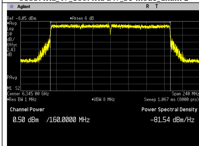
6345MHz_79_160MHz BW_be-mode_Chain 0
