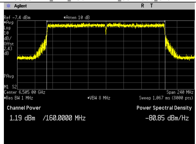
6505MHz_111_160MHz BW_be-mode_Chain 3
