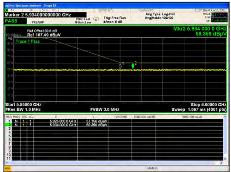
U-NII-2C 11n20 CH144 Peak
