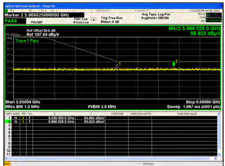
U-NII-2C 11n40 CH142 Peak
