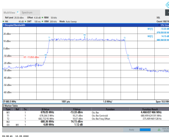
Band71-5MHz-QPSK-133297-25RB#0
