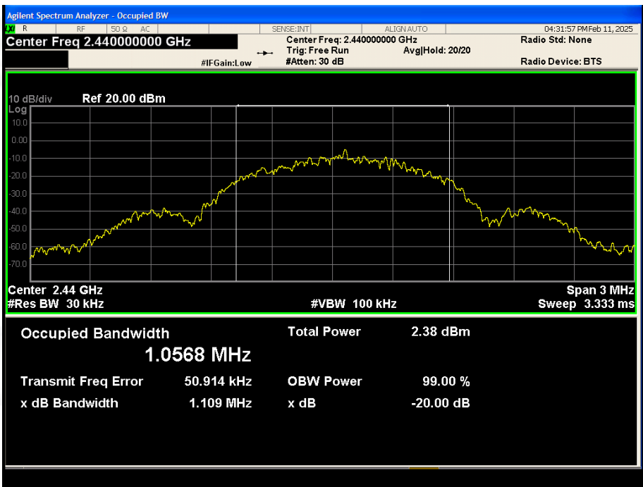
CH19: 2440MHz
