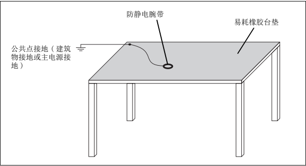
典型防静电台的安装
