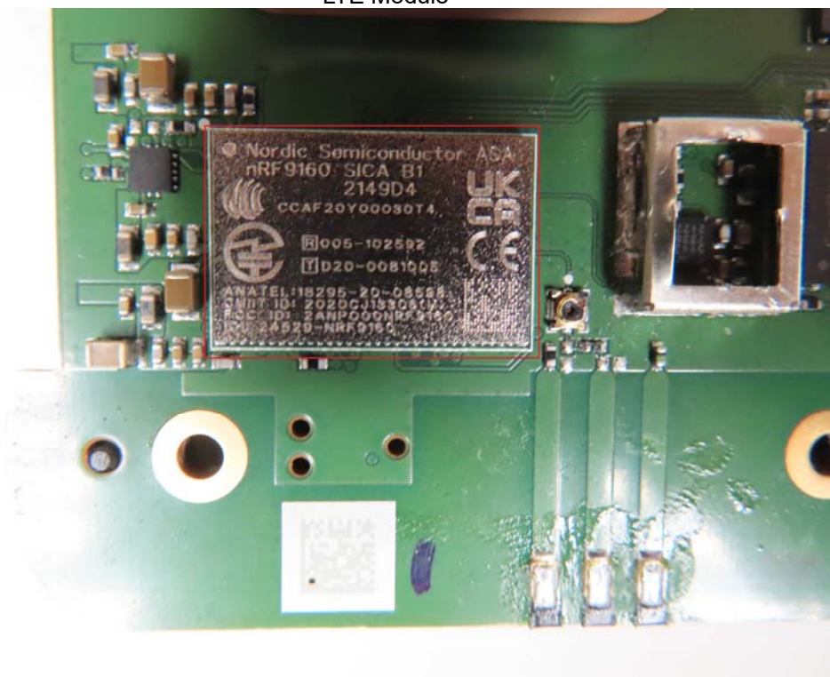
LTE Module
