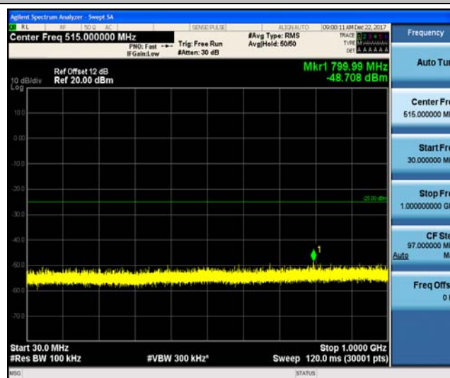
Band7_20MHz_QPSK_21100_1RB#0
