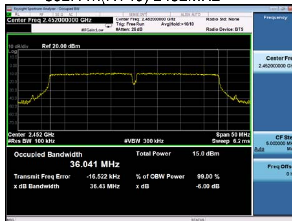
802.11n(HT40) 2452MHz
