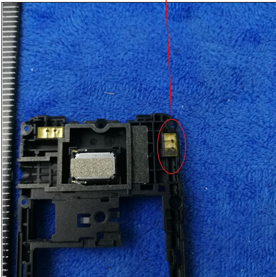
BT/WIFI/GPS Antenna
