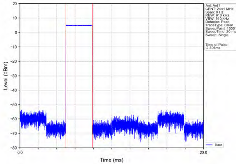
GFSK DH5 HOPP Ant1 NTNV
