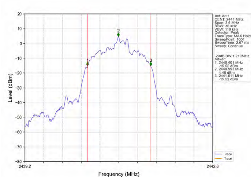
8DPSK 3DH5 MCH 2441MHz Ant1 NTN
