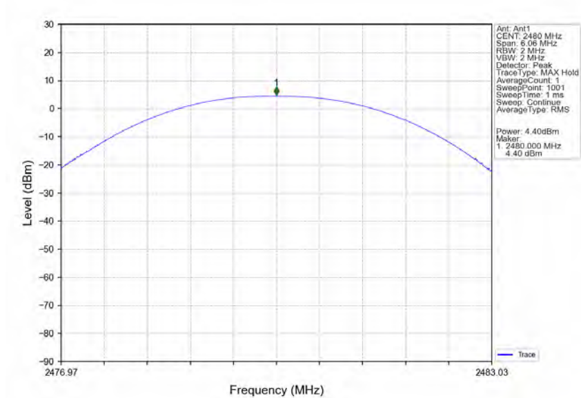
8DPSK 3DH5 HCH 2480MHz Ant1 NTNV
