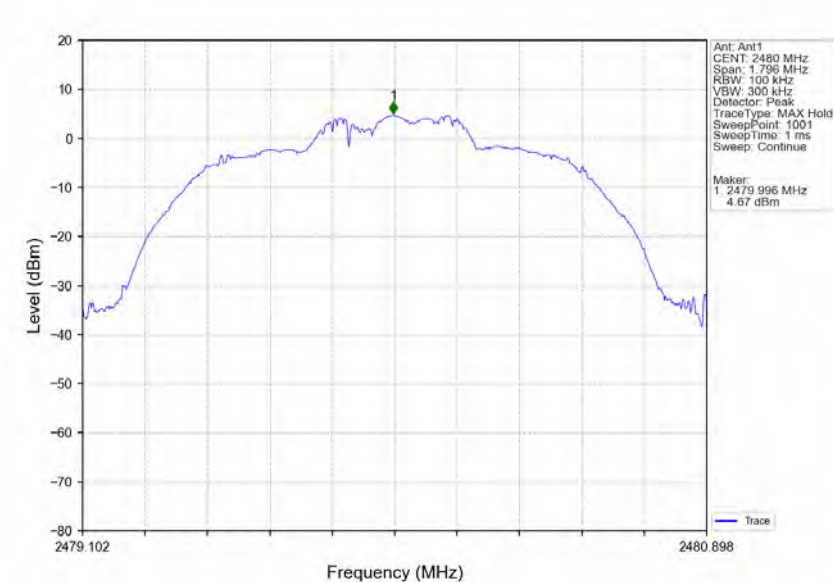
Pi/4DQPSK 2DH5 HCH 2480MHz Ant1 NTNV
