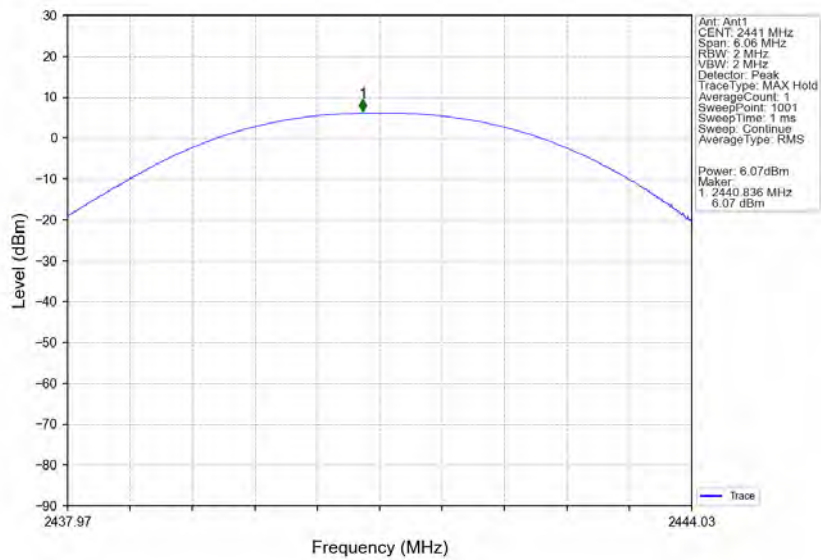
8DPSK 3DH5 MCH 2441MHz Ant1 NTNV
