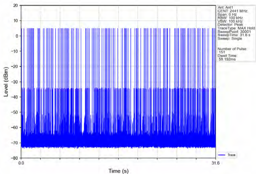
Pi/4DQPSK 2DH1 HOPP Ant1 NTNV
