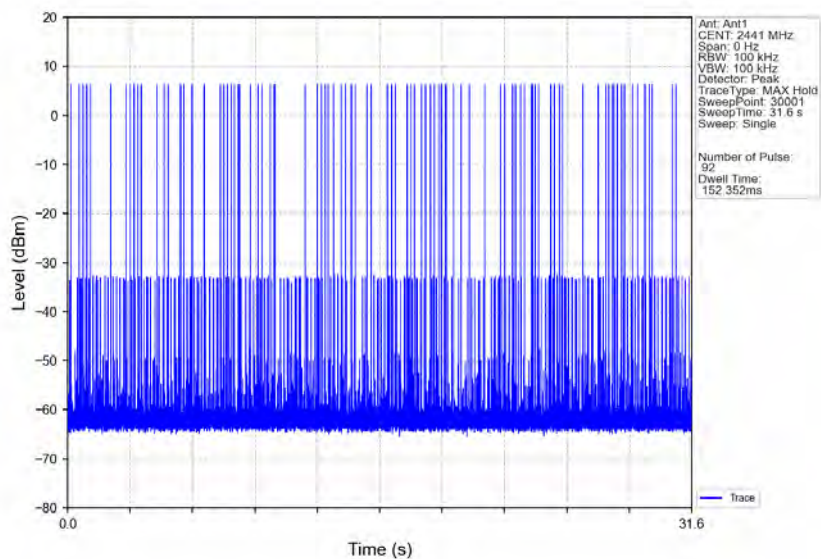
8DPSK 3DH3 HOPP Ant1 NTN
