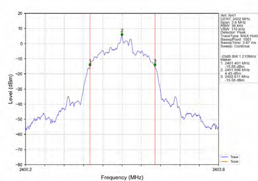
8DPSK 3DH5 LCH 2402MHz Ant1 NTN
