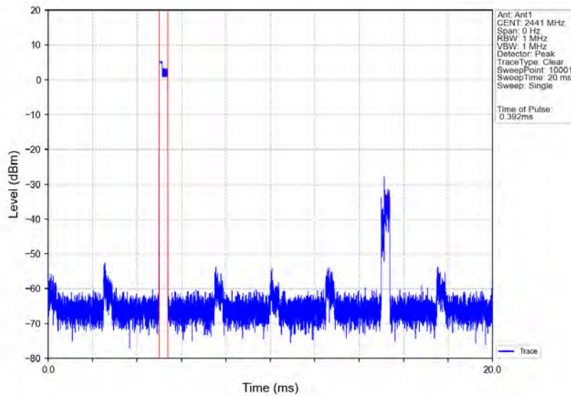
Pi/4DQPSK 2DH1 HOPP Ant1 NTNV
