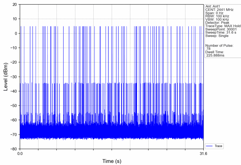
GFSK DH5 HOPP Ant1 NTNV
