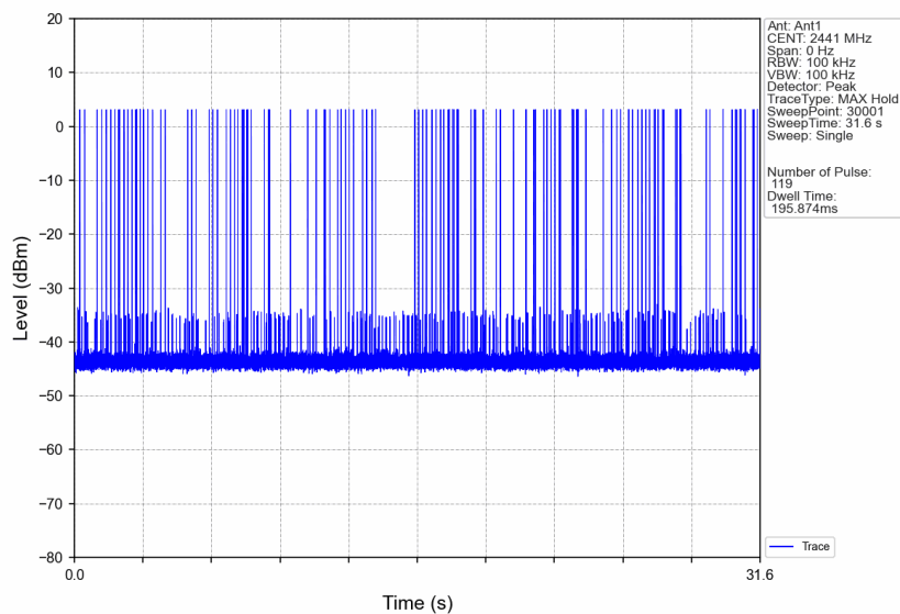
Pi/4DQPSK 2DH3 HOPP Ant1 NTN
