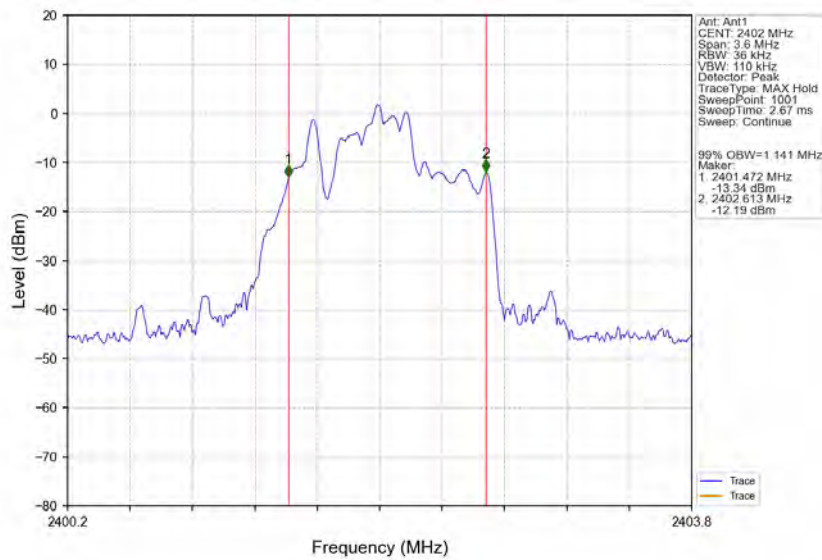
Pi/4DQPSK 2DH5 LCH 2402MHz Ant1 NTNV
