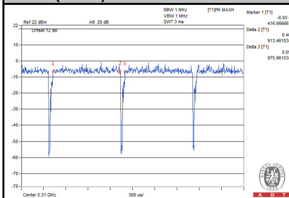
802.11n (40MHz)
