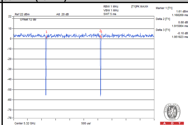
802.11n (20MHz)
