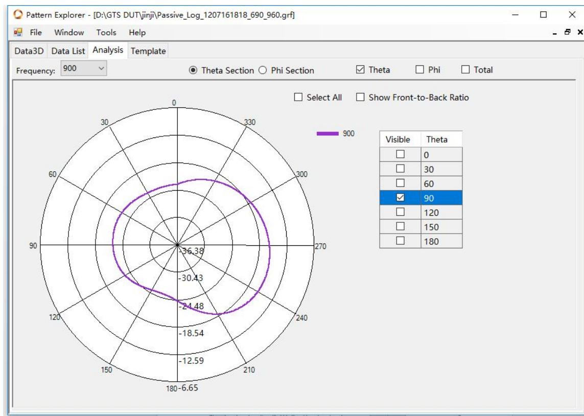
LTE B8 G900 W8 Theta=90deg
