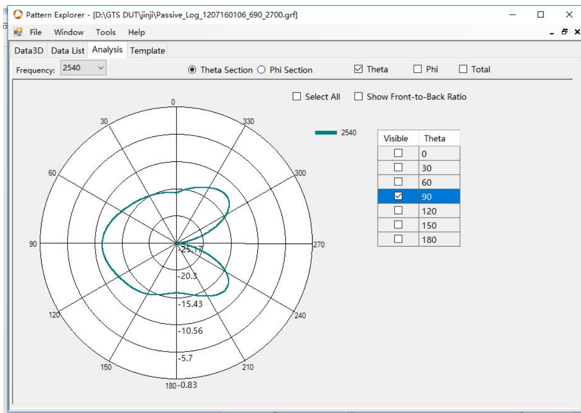
LTE B7 Theta=90deg
