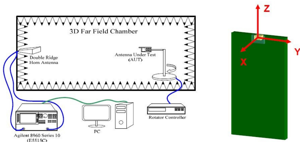
Fig.2 暗室示意图 FAR-field Chamber
