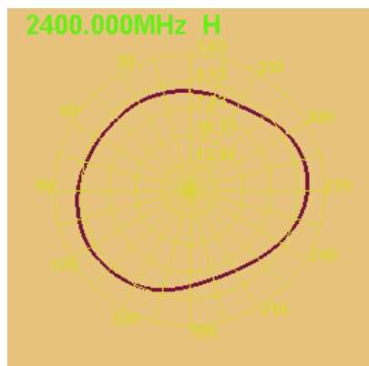
2D 增益模式 2D Gain Pattern (2400 MHz)
