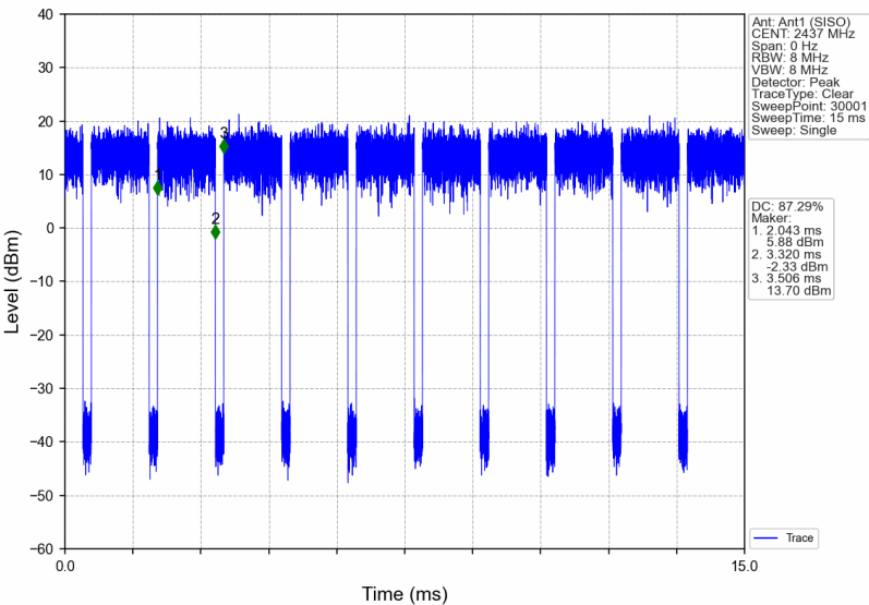
802.11n(HT20)_MCH_2437MHz_Ant1 (SISO)_NTNV
