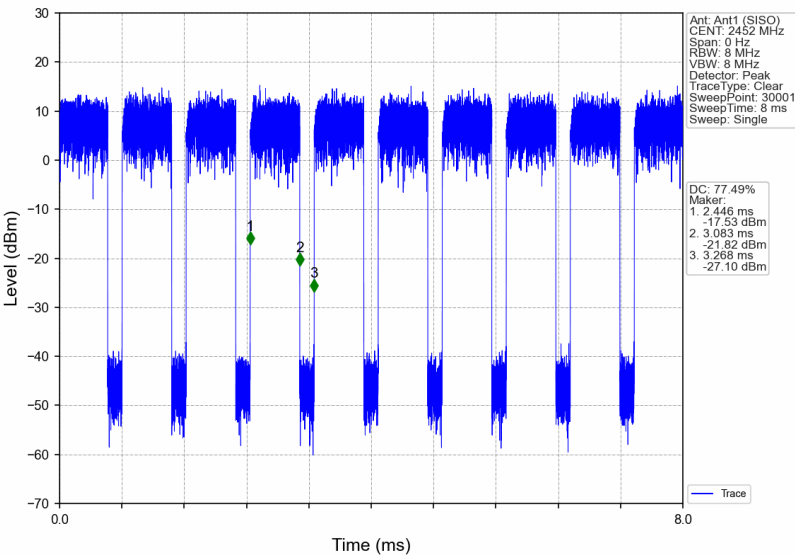
802.11n(HT40)_HCH_2452MHz_Ant1 (SISO)_NTNV
