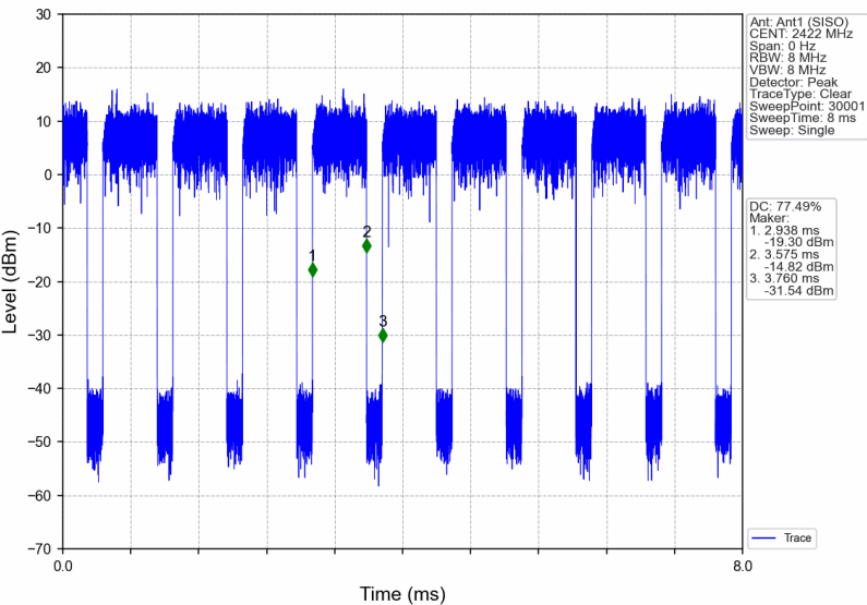
802.11n(HT40)_LCH_2422MHz_Ant1 (SISO)_NTNV
