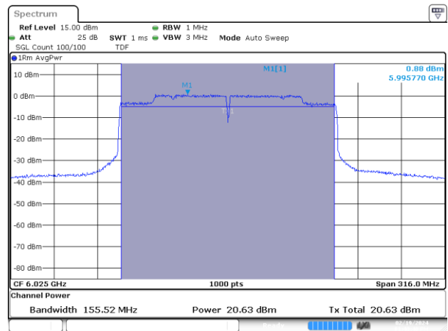
MIMO B-802.11ax/be-160MHz-Ch15-6025MHz-MCS0
