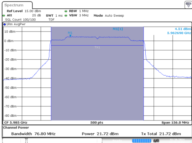
MIMO A-802.11ax/be-80MHz-Ch7-5985MHz-MCS0
