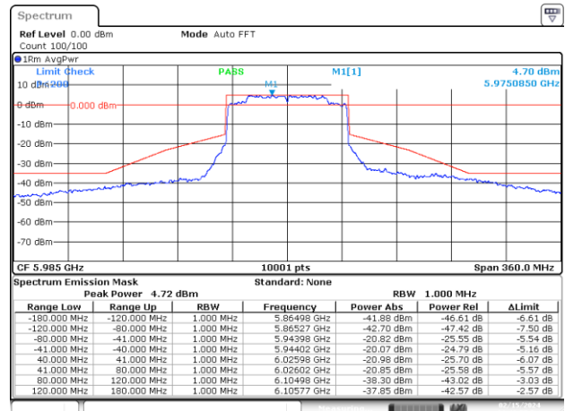
MIMO B-802.11ax/be-80MHz-Ch7-5985MHz-MCS0
