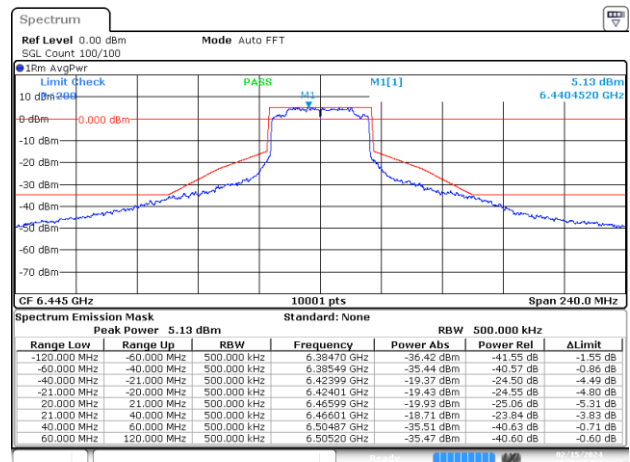
MIMO B-802.11ax/be-40MHz-Ch99-6445MHz-MCS0
