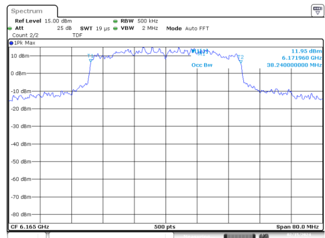
UNII5 SISO B 802.11ax/be40 ch43 6165MHz 99%
