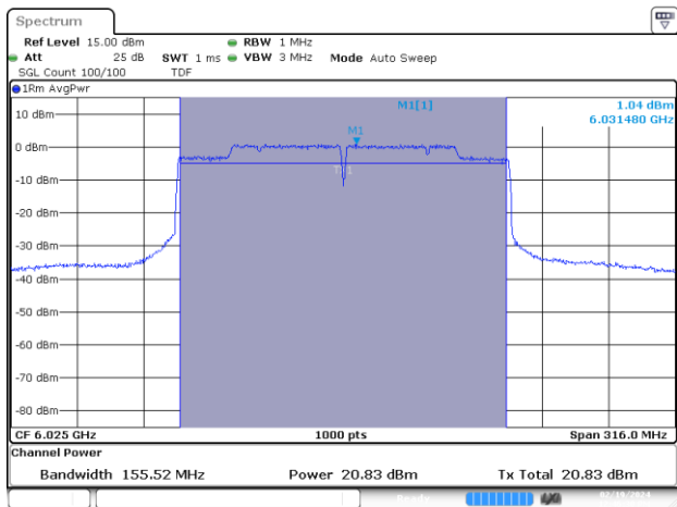
MIMO A-802.11ax/be-160MHz-Ch15-6025MHz-MCS0
