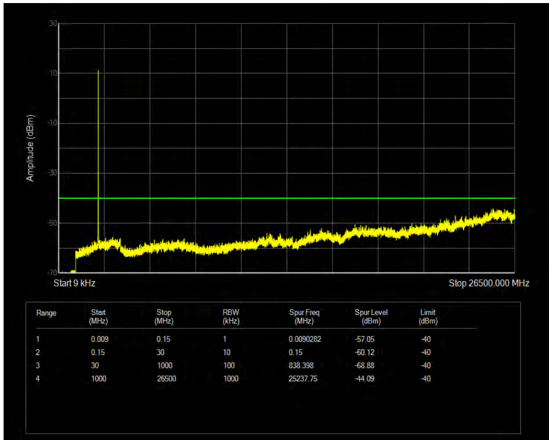
Band40(2305-2315) QPSK BW=10MHz Channel=38750 RB Size=1 Position=#0
