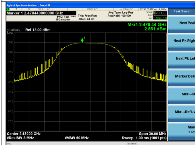
PWR-Zigbee 2480
