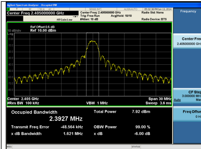
6dB BW TX-Zigbee 2405
