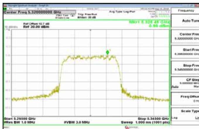
802.11a_20MHz_5320MHz
