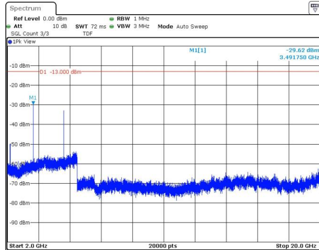
Band4-10MHz-QPSK-20350-50RB#0-Range1:30~1000MHz
