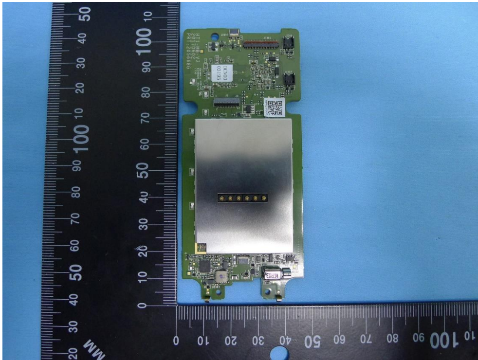
(5) EUT Photos
