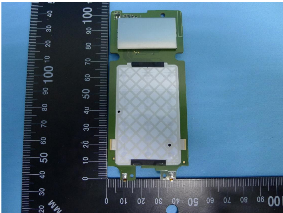
(6) EUT Photos
