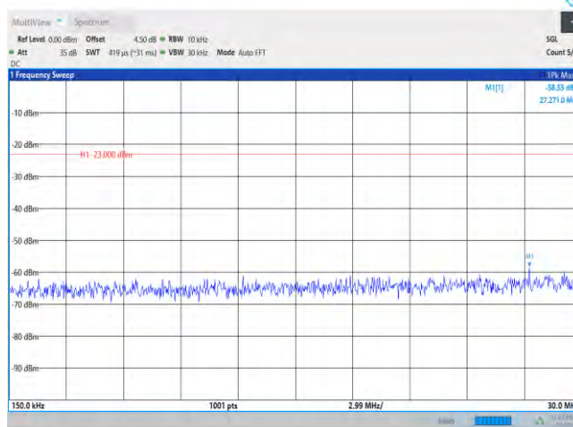
Band66-20MHz-QPSK-132072-1RB#0-Range2:0.15~30MHz
