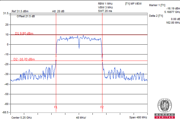
802.11ac (VHT160)_Chain 3 / CH50 (U-NII-2A)
