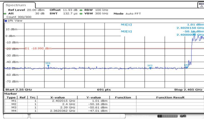
3DH5_Ant1_Low_Hop_2402
