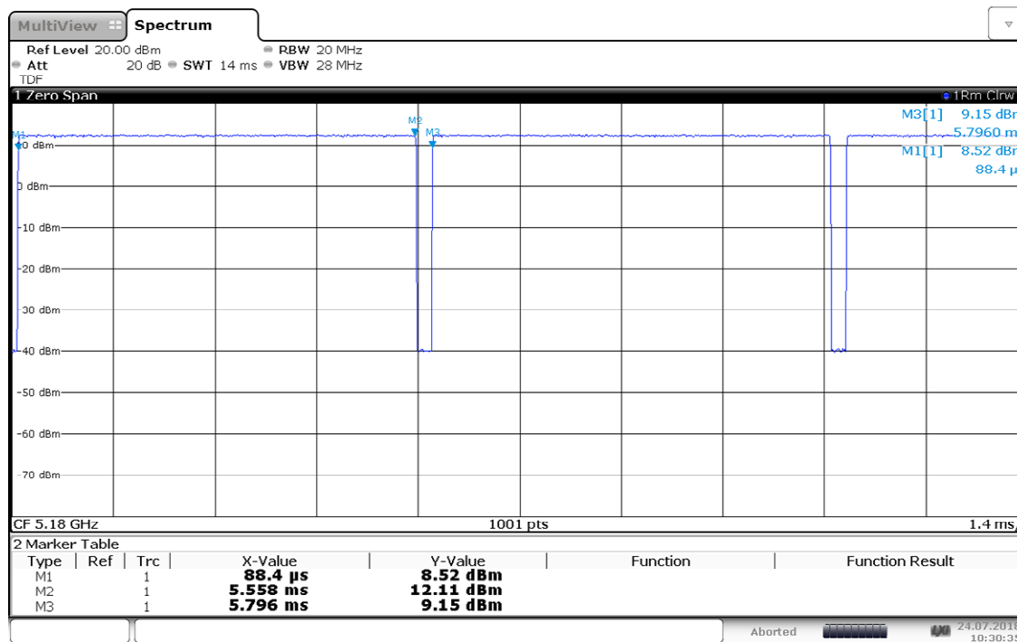
DC_36_a-mode_6Mbit
