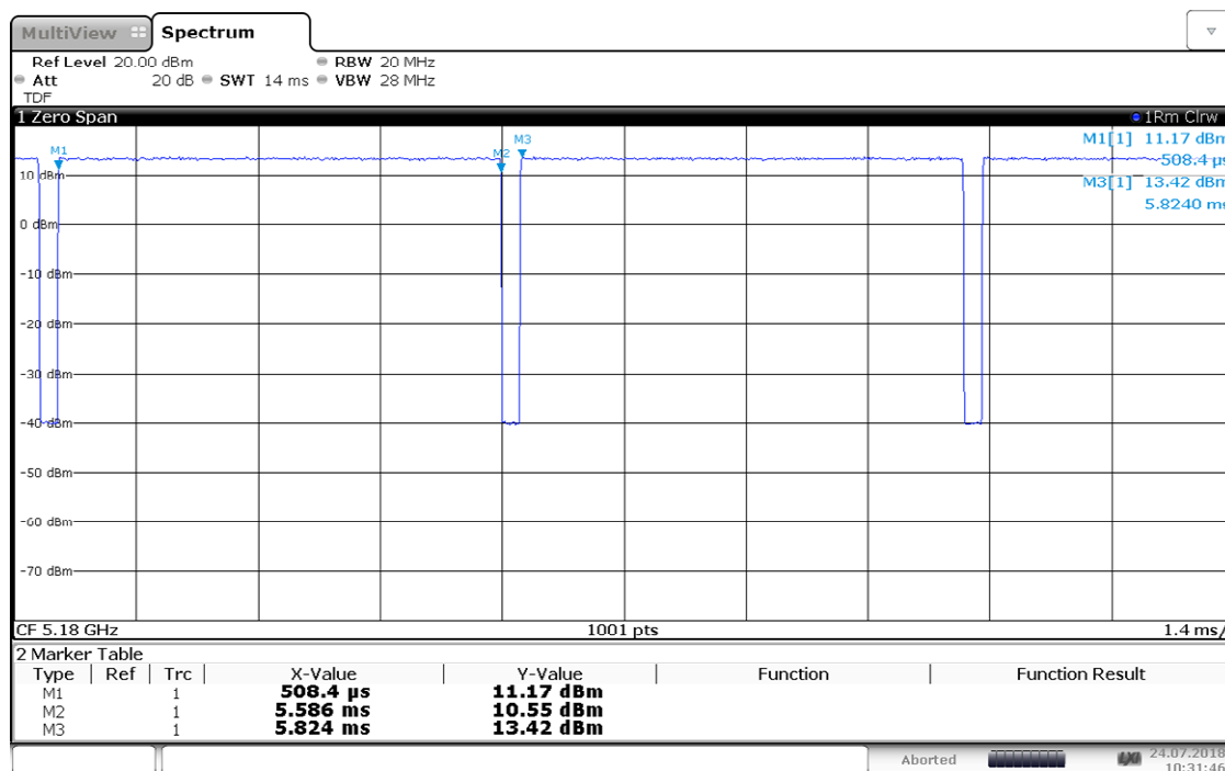
DC_36_n-mode_20M_MCS0
